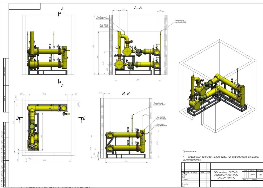
Реконструкция ГРП ОАО «Рязаньорггаз», г. Рязань
